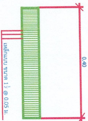
แปลนตะแกรงร่องระบายน้ำ SCALE NOT
