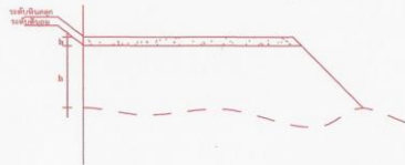
รูปตัดต้นทางดินถมและหินคลุก SCALE NOT
