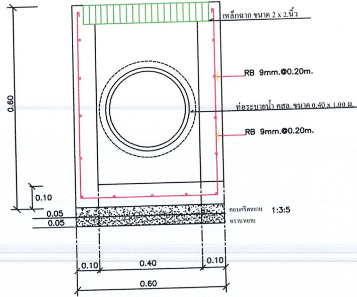
รูปตัดขยายบ่อพัก 2 SCALE not
